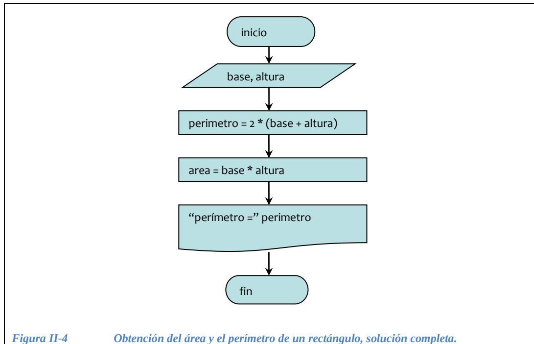
Figura II-4 Obtención del área y el perímetro de un rectángulo, solución completa.
