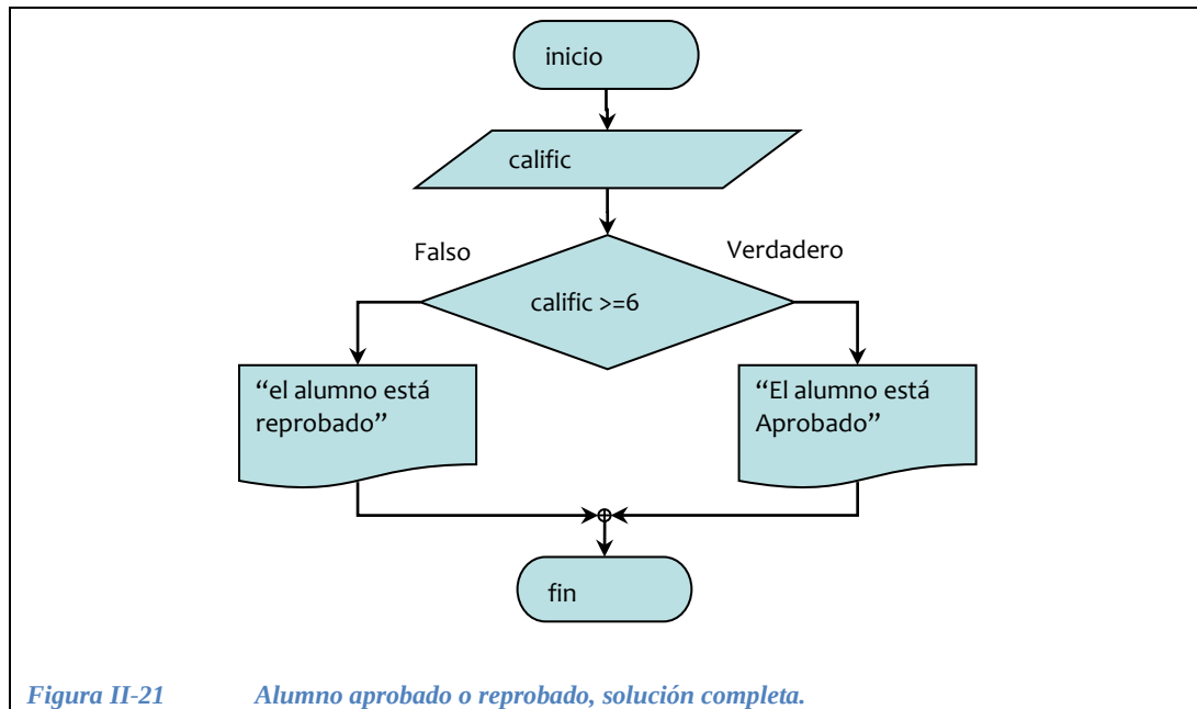
Figura II-21 Alumno aprobado o reprobado, solución completa.
