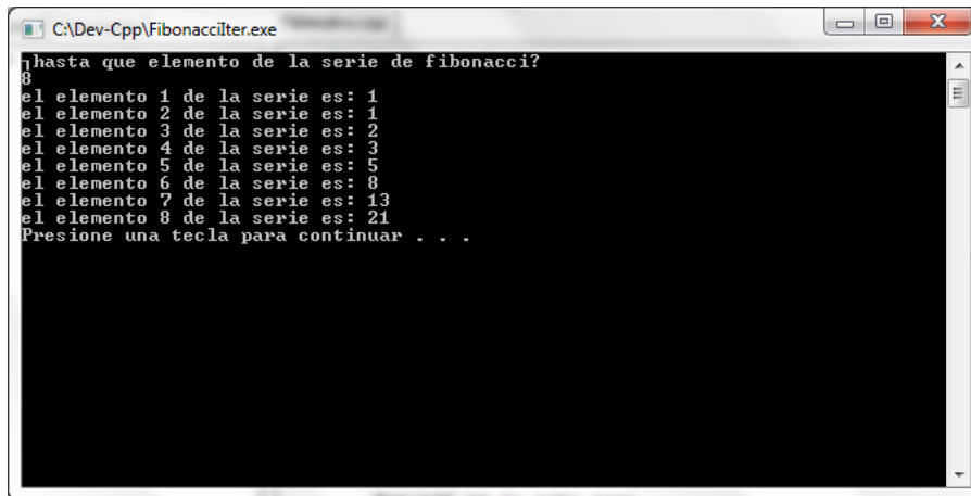
Figura VIII-5 Programa que obtiene los primeros 8 elementos de la serie de Fibonacci.
