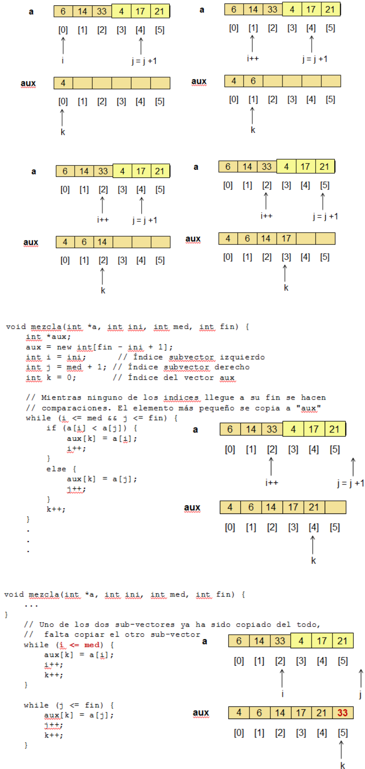
Figura VIII-9 Mezcla de subvectores.
