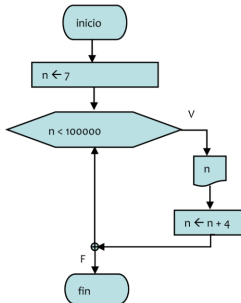
Figura II-52 Algoritmo para escribir la serie 7, 11, 15, 19, ... mientras los números sean menores a 100,000.
