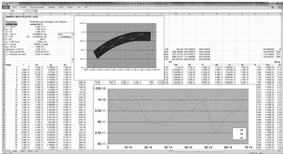
FIGURA 1. RESULTADO TÍPICO DE LA DINÁMICA MOLECULAR EN LA HOJA DE CÁLCULO. EL TOTAL DE COLUMNAS ES DE 45, CON MÁS DE 2000 RENGLONES DE ITERACIÓN. LAS GRÁFICAS MUESTRAN LAS POSICIONES DE UNO DE LOS ÁTOMOS EN EL ESPACIO O EN FUNCIÓN DEL TIEMPO
