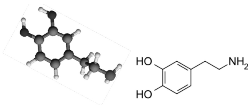
FIGURA 2. DISTINTAS REPRESENTACIONES DE LA DOPAMINA
