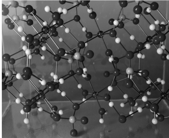
FIGURA 2. MODELO DE "BOLAS Y ALAMBRES". LAS ESFERAS REPRESENTAN A LOS DIFERENTES TIPOS DE ÁTOMOS; LOS ALAMBRES, A LOS ENLACES ENTRE ÁTOMOS
