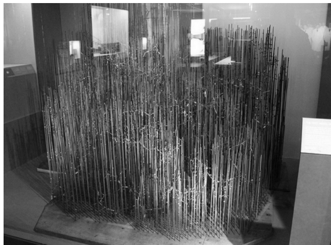
FIGURA 1. MODELO DE ALAMBRES DE LA MIOGLOBINA
